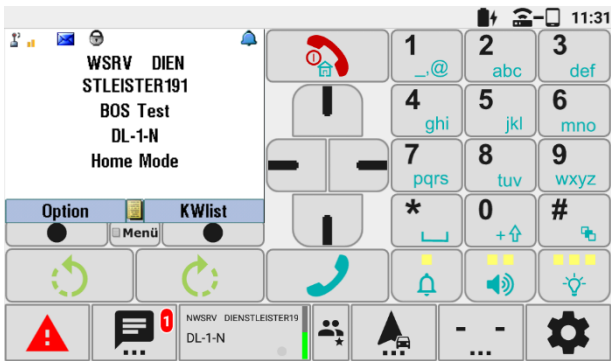
Konsolenbedienung Motorola
